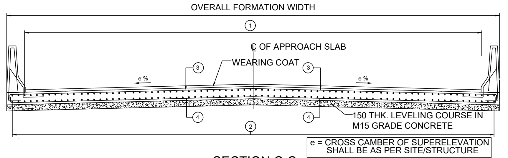
SECTION C-C (SCALE:-1:50)
