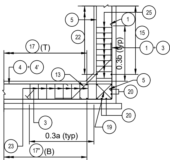
DETAIL-1 (SCALE-1:40)
