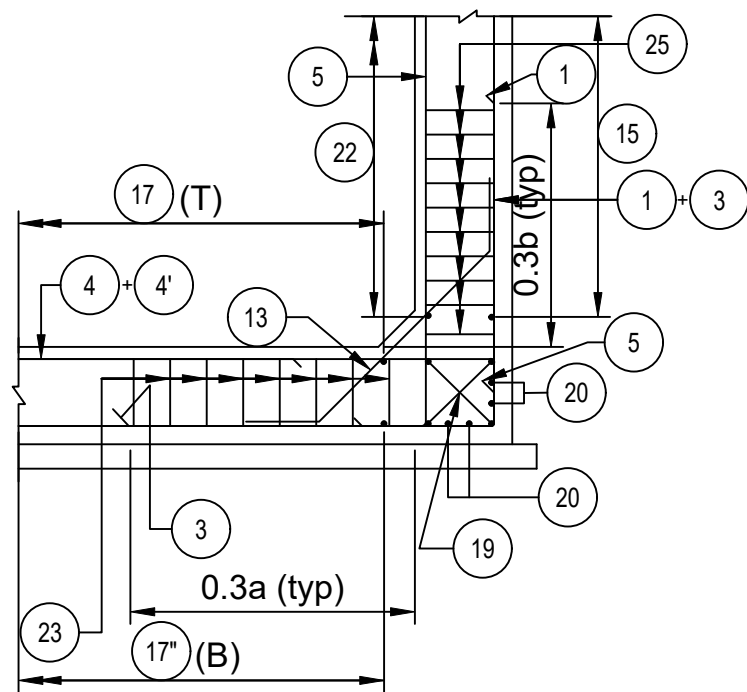
DETAIL-1 (SCALE-1:40)
